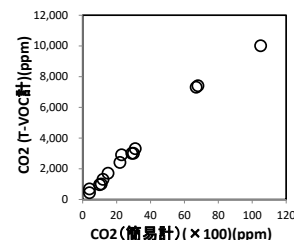
図2 CO 2 測定値の比較
