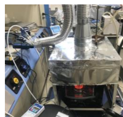
図1 作製した燃焼実験装置
