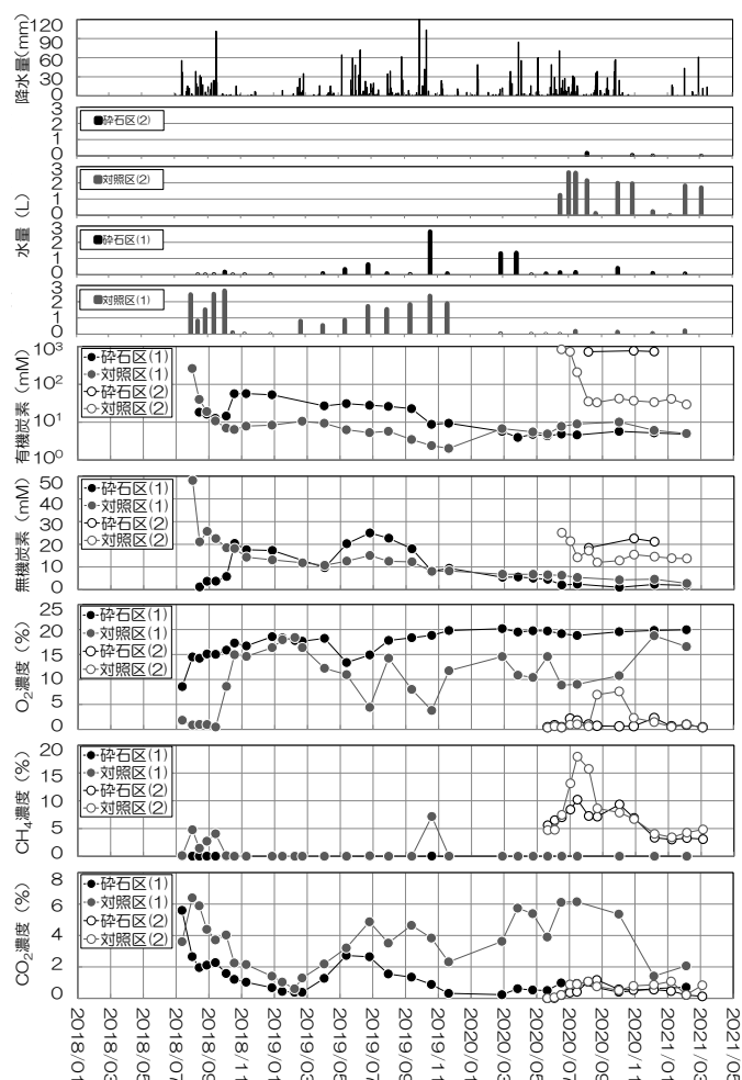
図1 降水量、浸透水量、水質、ガス濃度の経月変化
