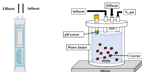
図1 試験装置図
