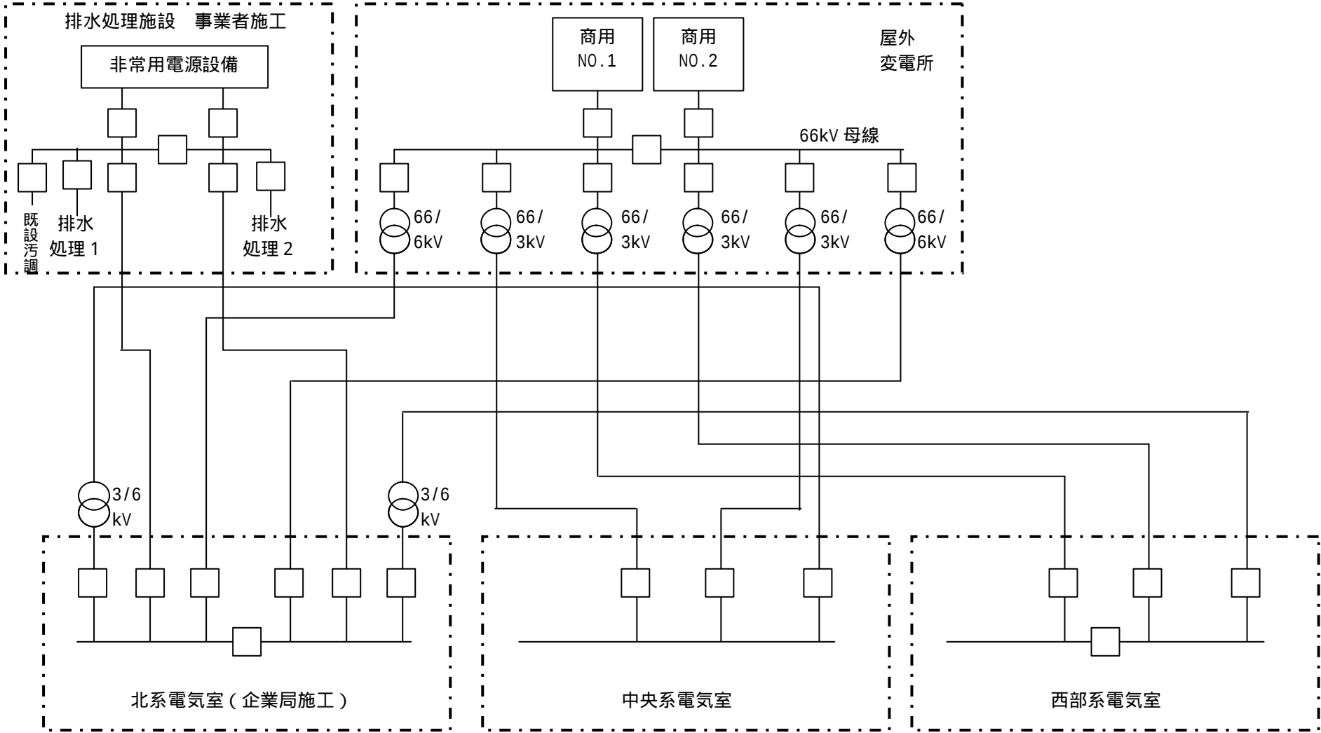
排水処理施設・非常用電源施設電源系統図
